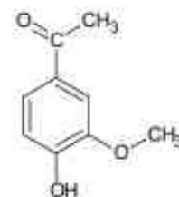
acetovanillone
